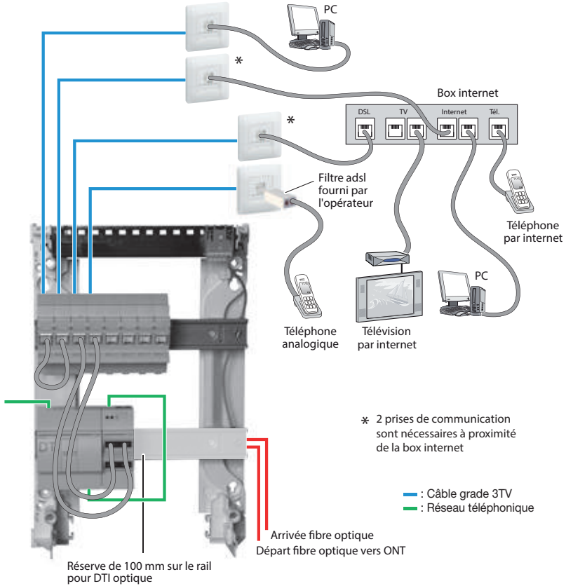
Sur goulotte
