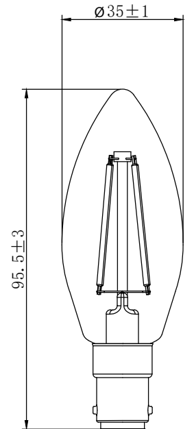
B35 avec culot B15
