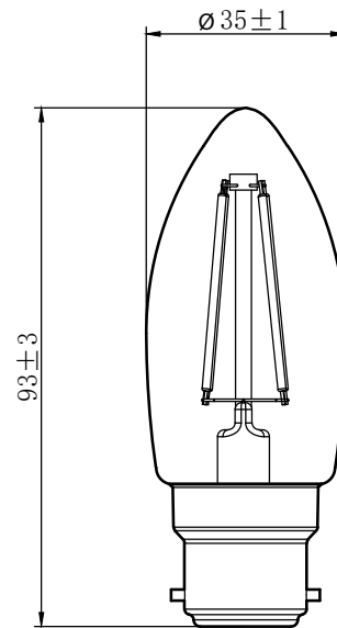
B35 avec culot B22
