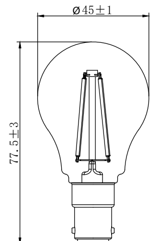
P45 avec culot B15
