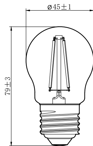
P45 avec culot E27
