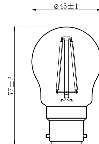
P45 avec culot B22
