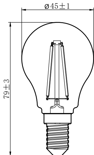
P45 avec culot E14
