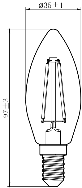
B35 avec culot E14
