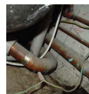
Liaison équipotentielle
